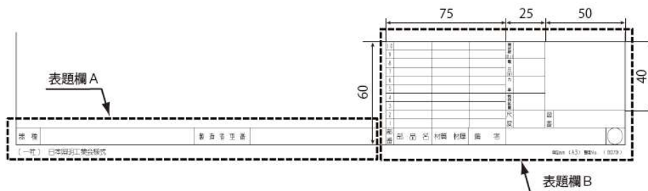
図 2—様式の表題欄寸法
